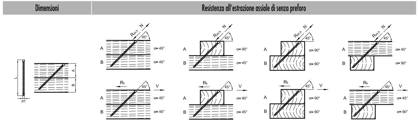
Valore caratteristico della portata della connessione R_k secondo ETA-11/0024
