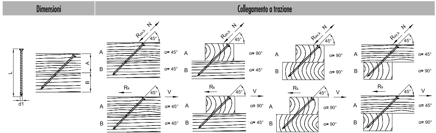
Valore caratteristico della portata della connessione R_{ox,k} e/o R_k secondo ETA-11/0024
