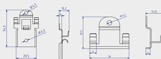
Clip per facciate Rhombus
