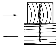
Collegamento montante/traversa
