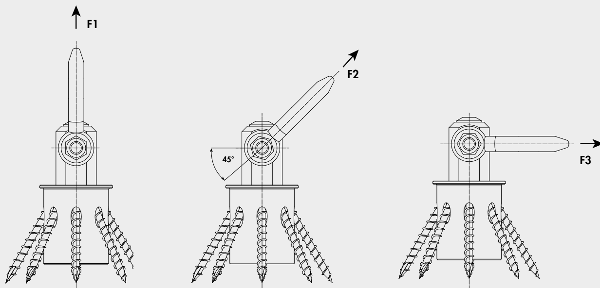
L'ancoraggio di sollevamento Mini insieme ai bulloni di supporto sferici.
